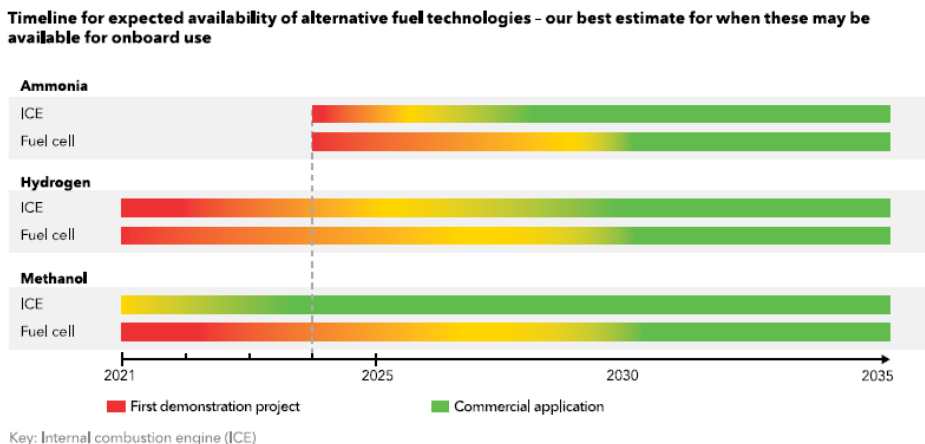
Ilusiliaq 24. Umiarsuit angallannerini teknologiinut toqqartukkanut pissarsiarineqarsinnaasunut inerisimasunullu takussutissiaq: (DNV, 2021)
